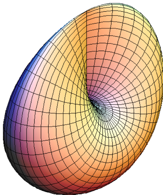
Exemple de cross-cap
